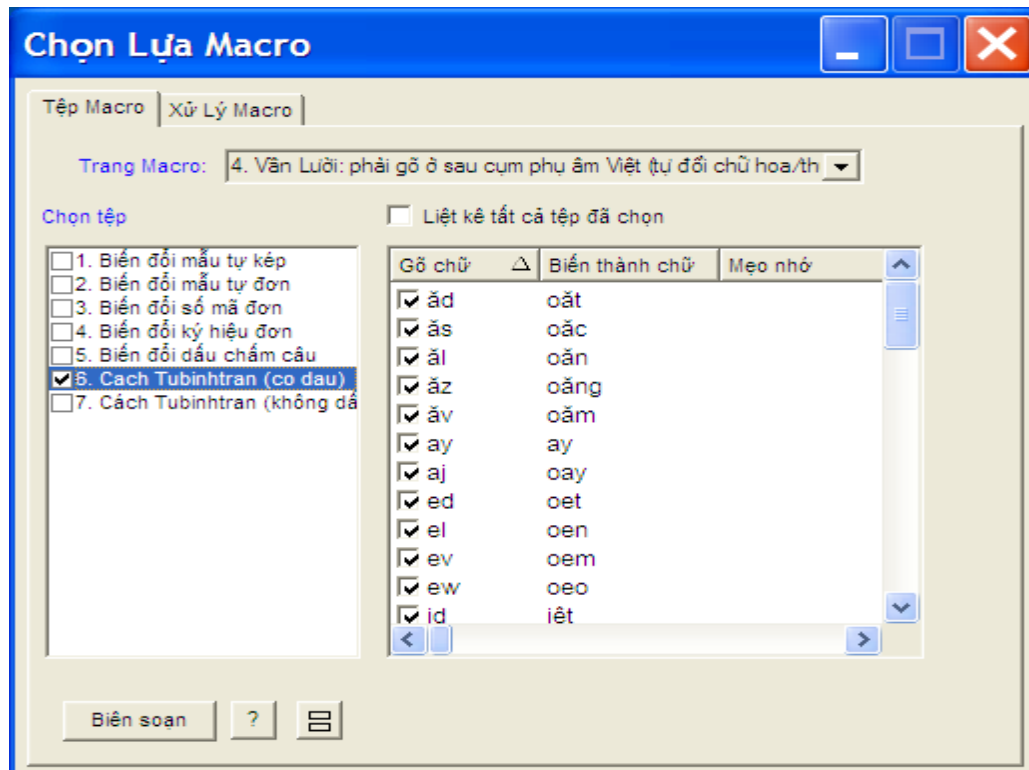
Hình 16: Khung "Chọn Lựa Macro" khi dùng cách gõ tắt Tubinhtran có dấu.
