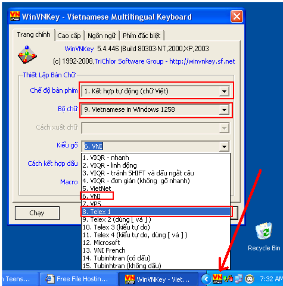
Hình 13: Điều chỉnh WinVNKey để gõ chữ Việt trong Audition.
