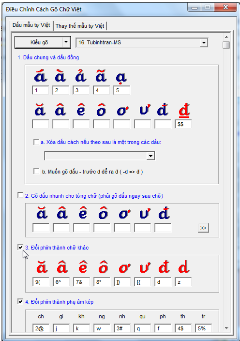
Hình 5: Bảng “Điều chỉnh Cách Gõ Chữ Việt” cho kiểu gõ Tubinhtran-MS.
